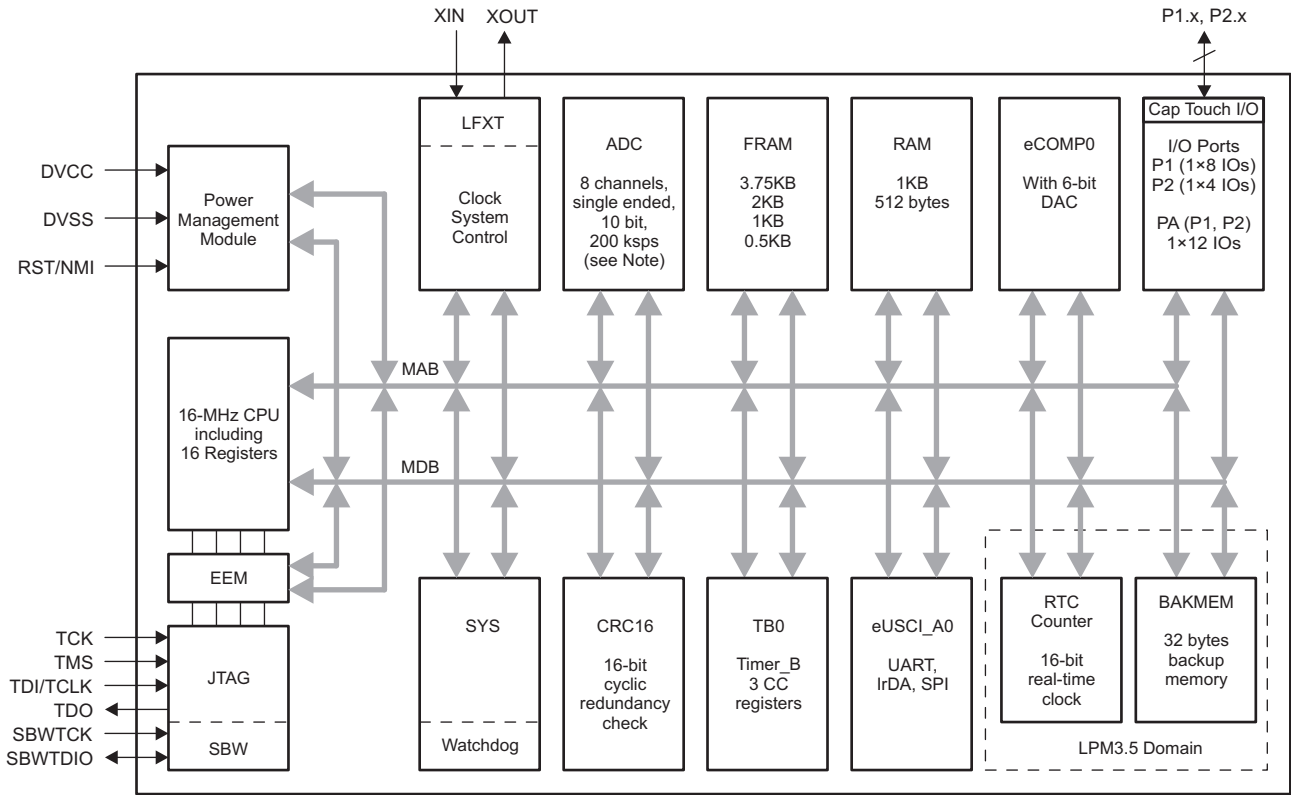
图 1-1. 功能框图
