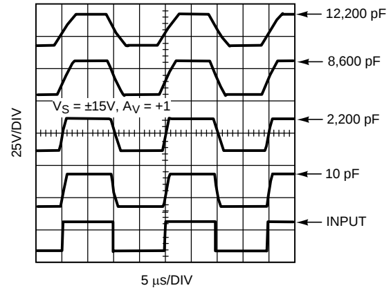
图 50. 大信号阶跃响应
