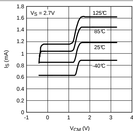
图 28. I_S 与 V_{\text{CM}} 间的关系 (LM7321)
