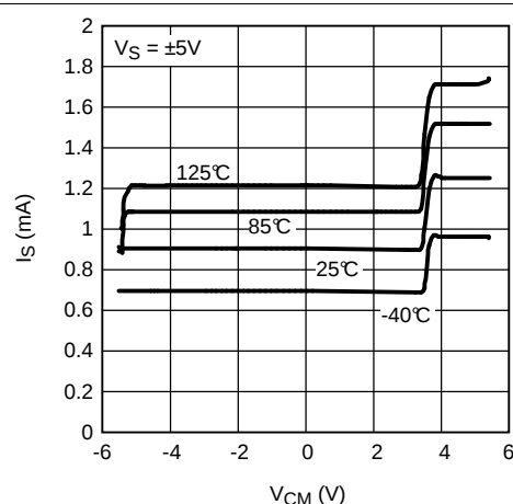
图 30. I_S 与 V_{\text{CM}} 间的关系 (LM7321)
