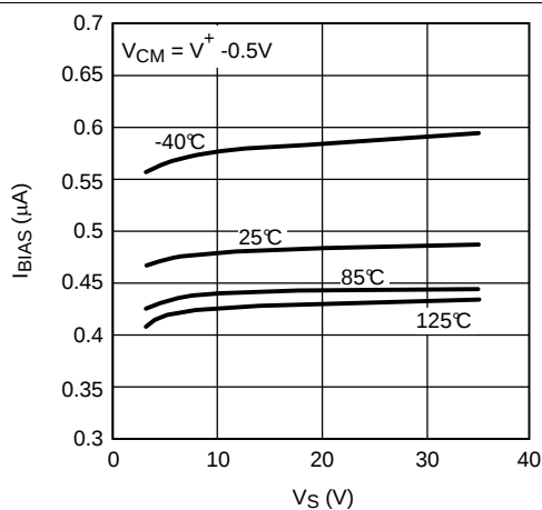
图 27. I_{\text{BIAS}} 与 V_S 间的关系
