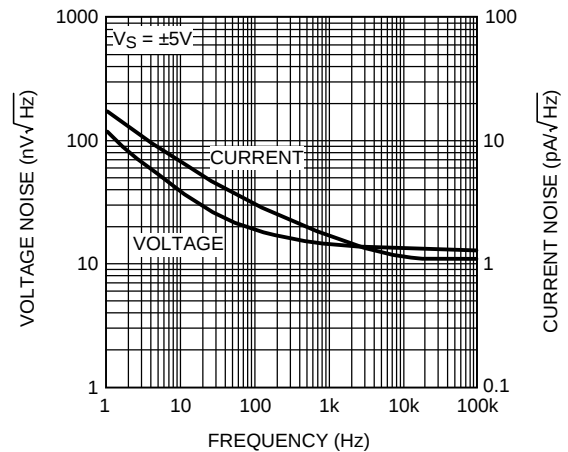
图 52. 输入基准电压噪声密度与频率间的关系
