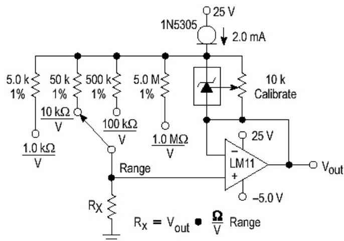
Fig 17. Liner ohmmeter
