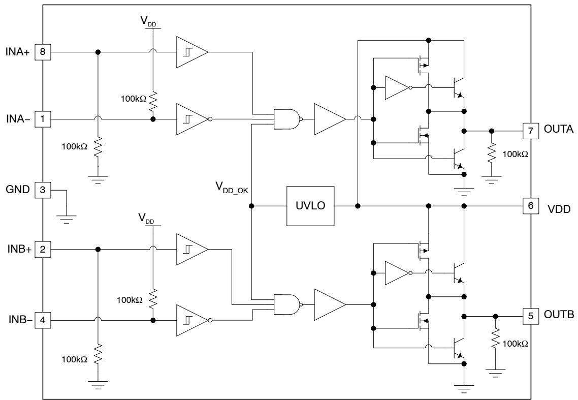
图 7. FAN3228 框图
