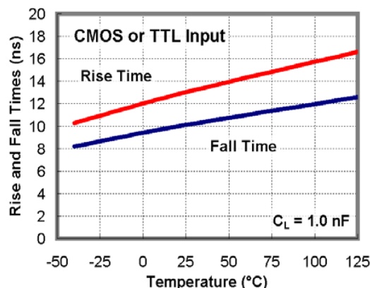
图 39. 上升/下降时间与温度的关系
