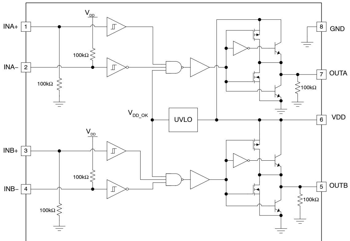
图 8. FAN3229 框图
