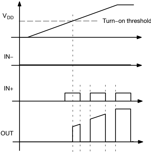
图 52. 同相启动波形
