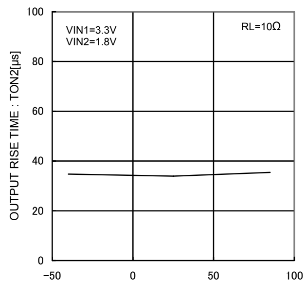
Figure 25. Output rise time2
