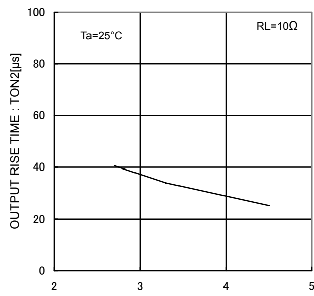
Figure 24. Output rise time2
