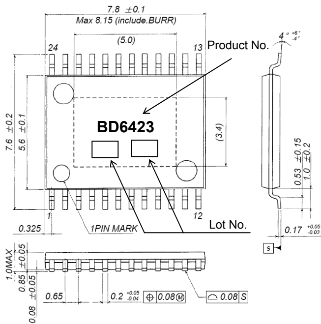
HTSSOP-B24 (Unit:mm)
