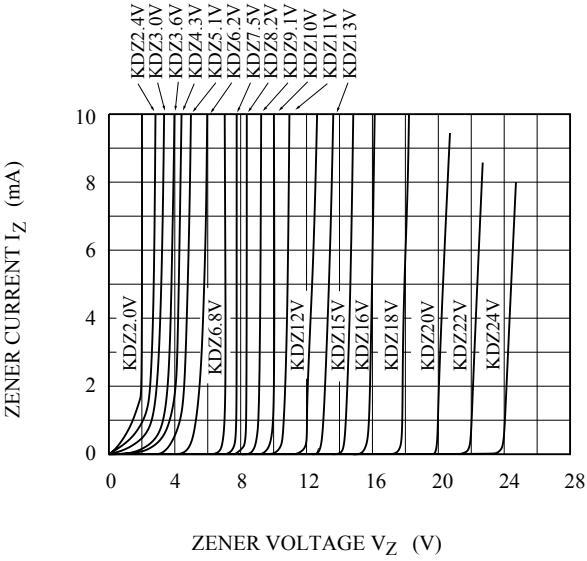
I_Z - V_Z
