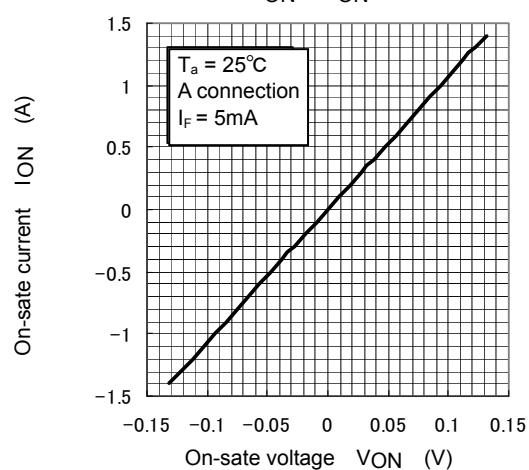
I_{ON} - V_{ON}
