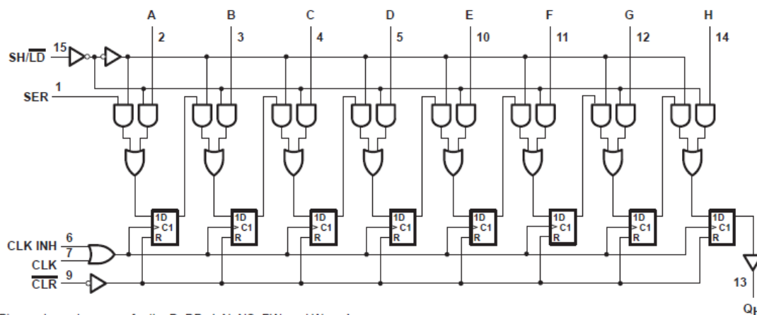
功能框图
