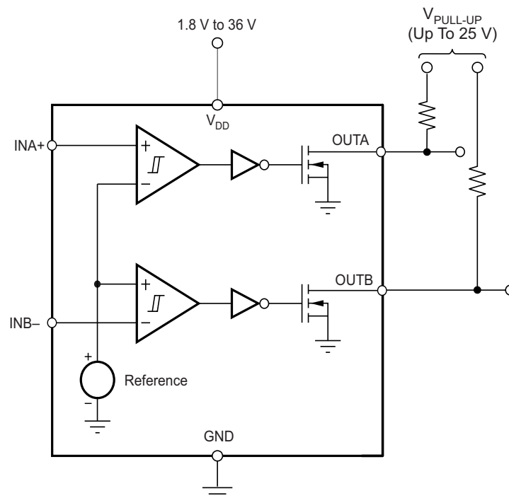
简化框图
