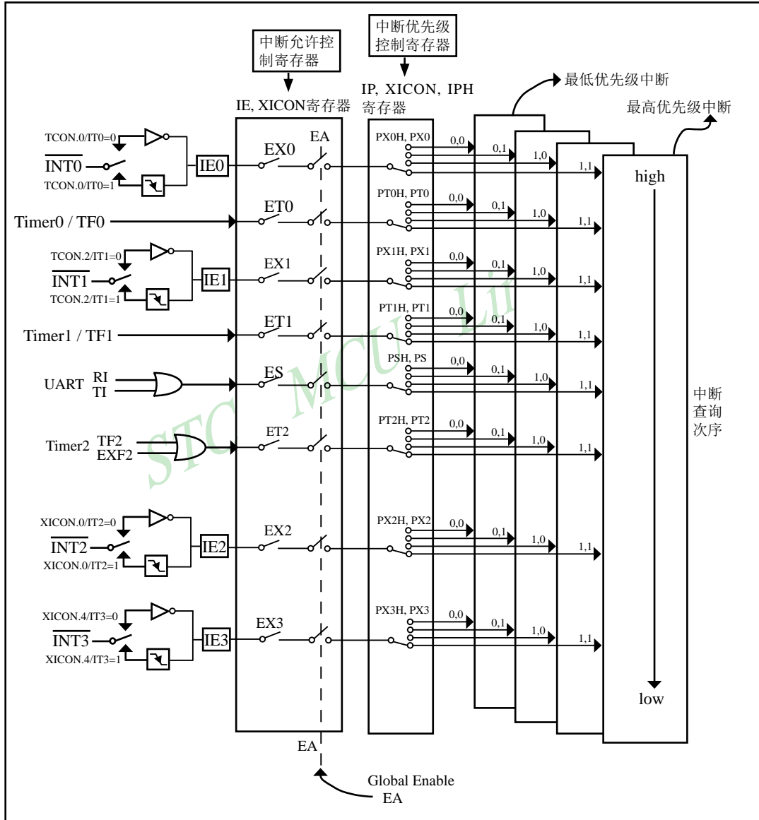
图6-1 STC90C51RC/RD+系列中断系统结构图
