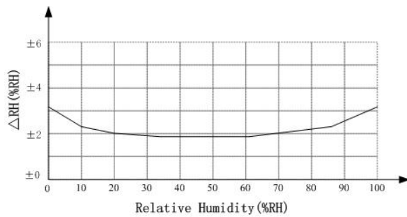
图 2: 25℃时 AM2322 的相对湿度最大误差
