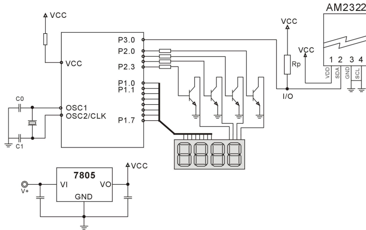
图 19： AM2322 单总线典型电路
