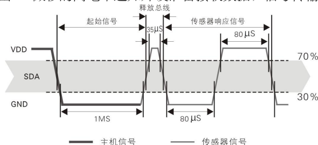
图 22: 单总线分解时序图
