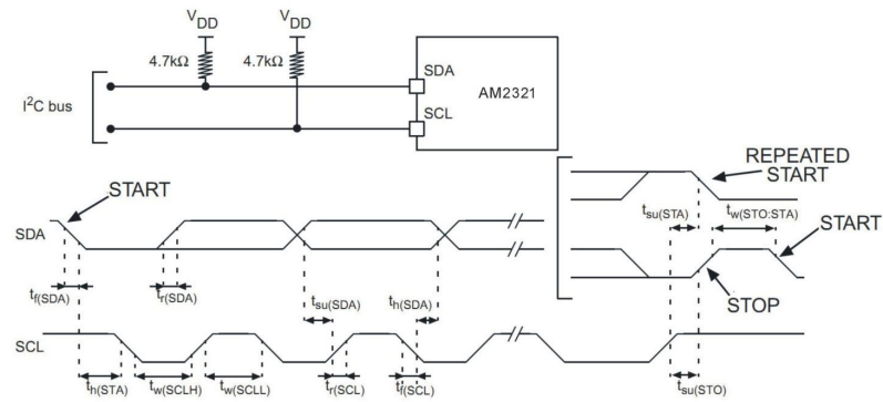
图 13: AM2322 典型的 I2C 总线应用电路和时序图
