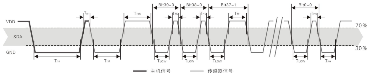
图 21: AM2322 单总线通信时序
