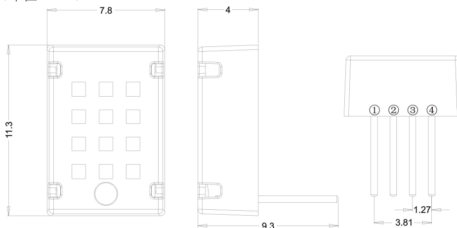
图1 AM2322 外形尺寸
