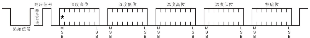
图 20： AM2322 单总线通信协议
