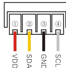
图 4: AM2322 接线图
