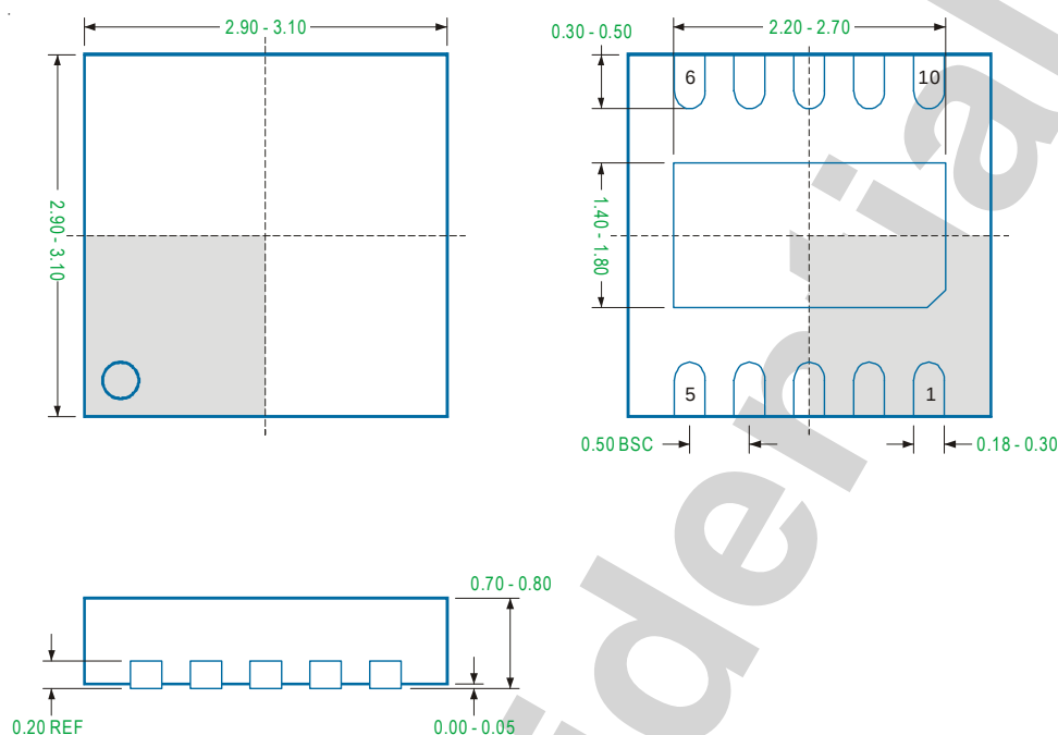
WDFN3x3 - 10L
