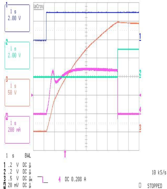
Fig 1. VBAT=3.0V
