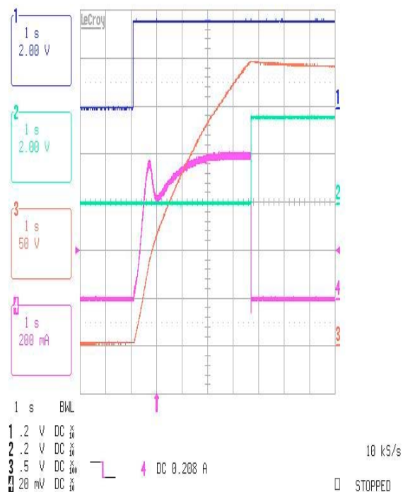
Fig 2. VBAT=3.6V
