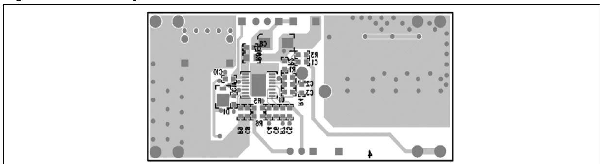
Figure 25. Bottom layer
