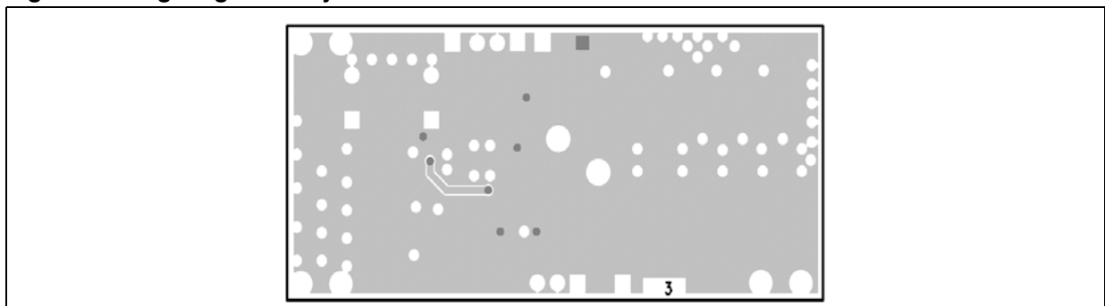
Figure 25. Bottom layer
