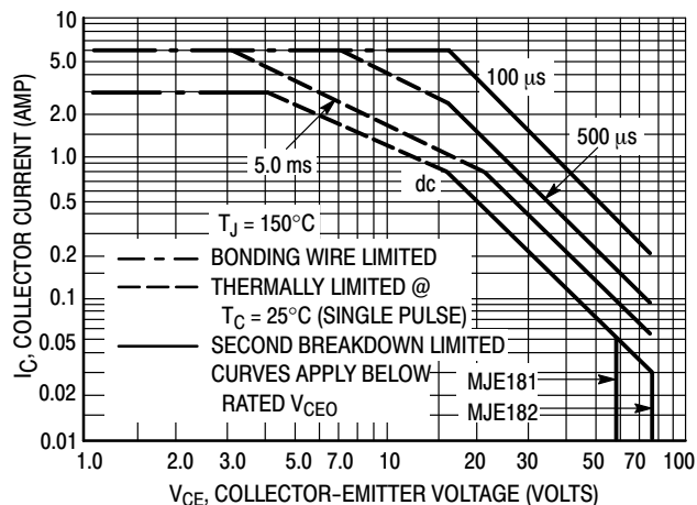
Figure 6. MJE181, MJE182
