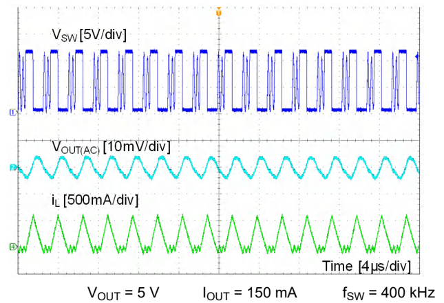
图 9-3. DCM Mode
