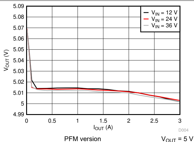
图 7-5. Load Regulation
