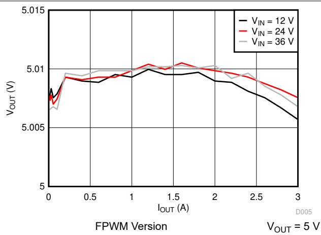
图 7-6. Load Regulation
