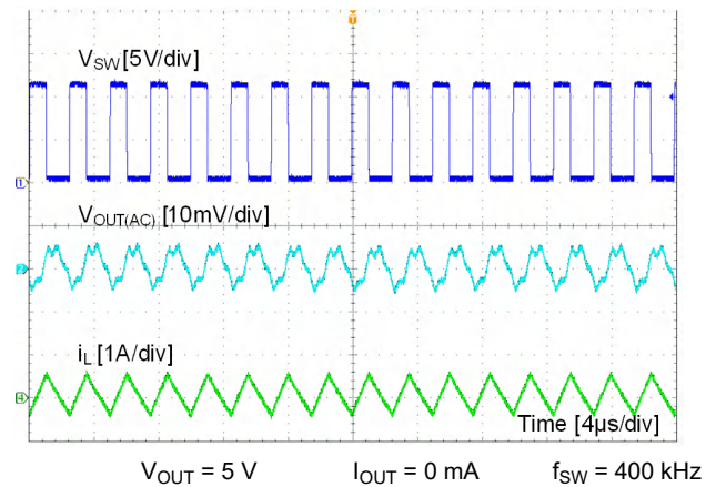
图 9-5. FPWM Mode
