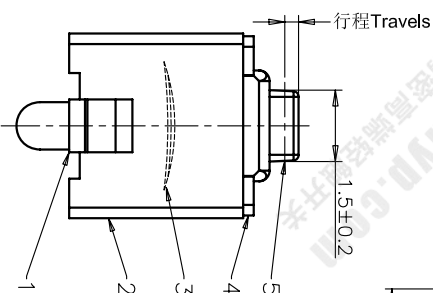
安装尺寸图
