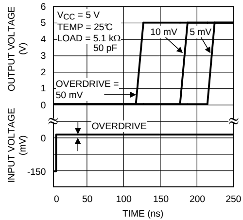
图 14. 传播延迟与过驱电压间的关系
