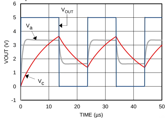
图 25. 方波振荡器输出波形
