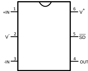
SOT-23 的引脚功能
