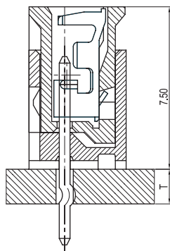
PCB ASS'Y
