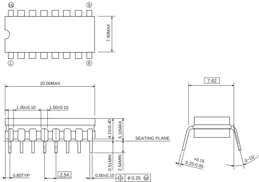
DIP16-G-300-2.54
