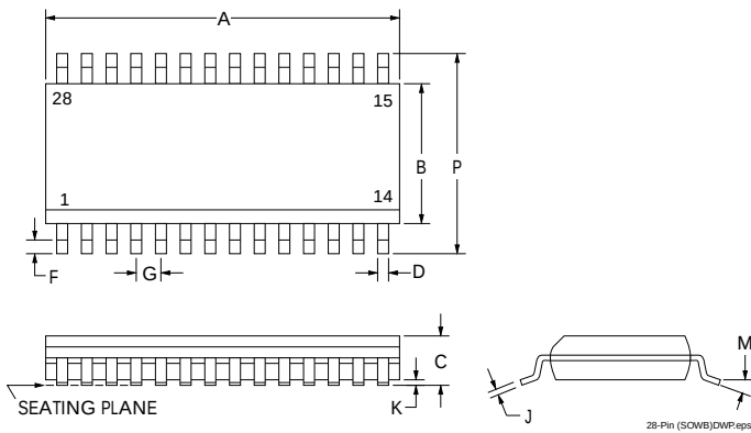
SOWB (28-Pin)
