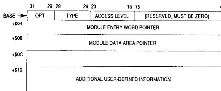
Figure 9-10. Module Descriptor Format
