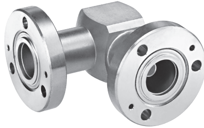
7/8" EIA flange
