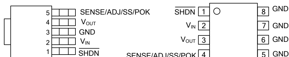
TO-252-4/TO-252-5/TO-263-5
