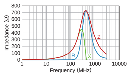
MMZ1608F030BTA00
