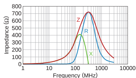
MMZ1608Q102BTA00
