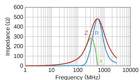
MMZ1608D241CTA00
