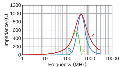
MMZ1608F470BTA00
