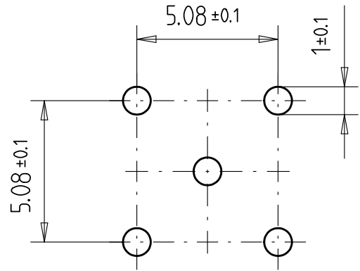
Bohrbild
