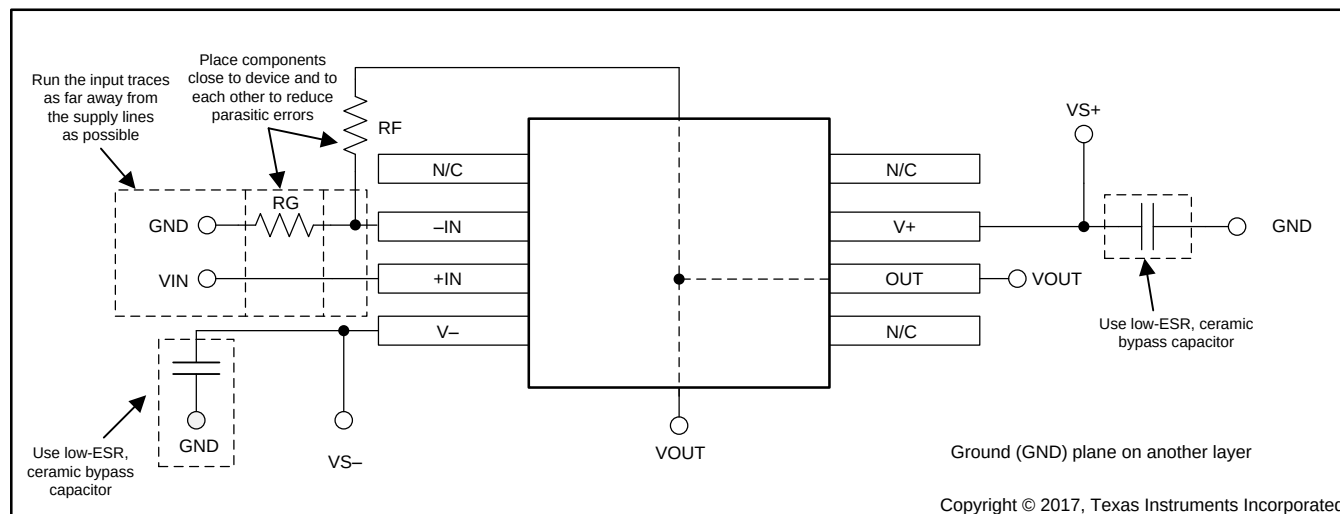
图 48. Layout Example
