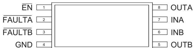
TSSOP-8
