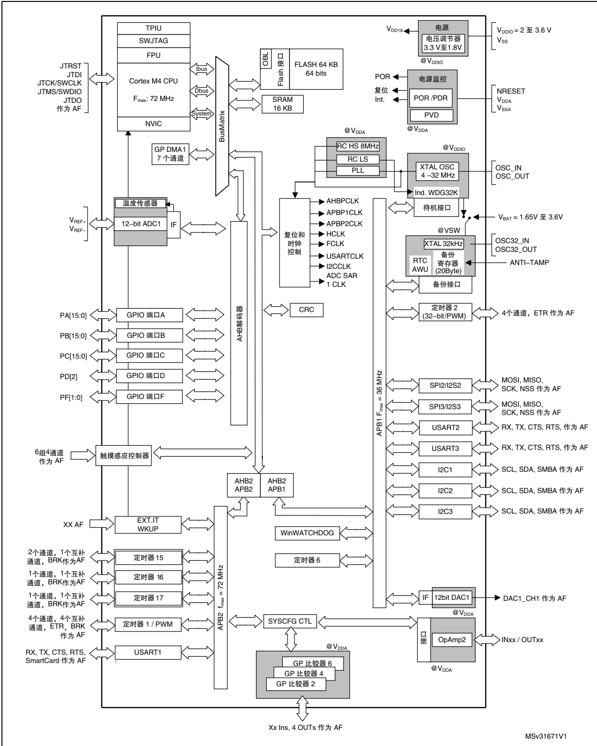
图 1. STM32F301x6/8 框图
