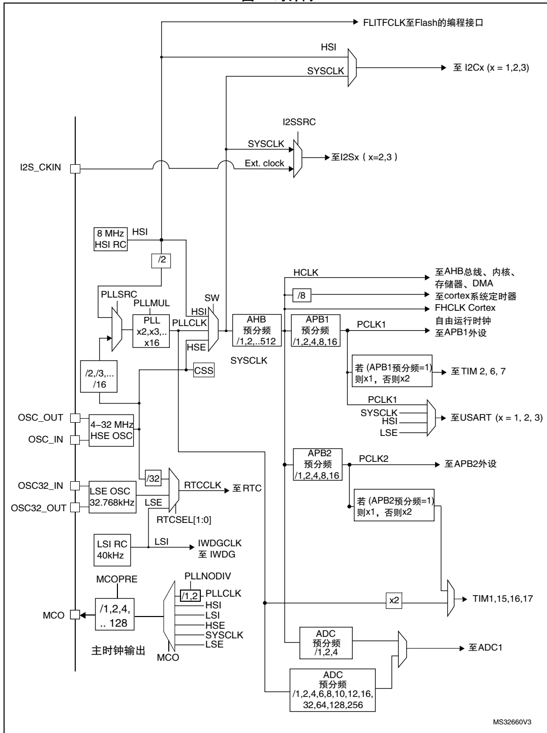
图 2. 时钟树
