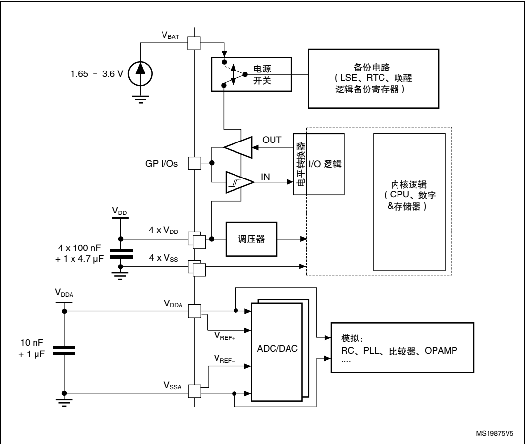
图 11. 电源方案
