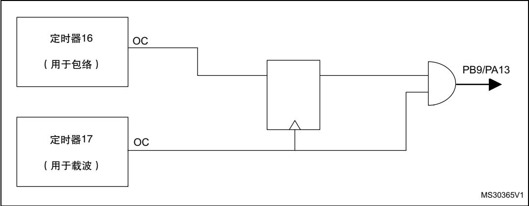
图 3. 红外发射器
