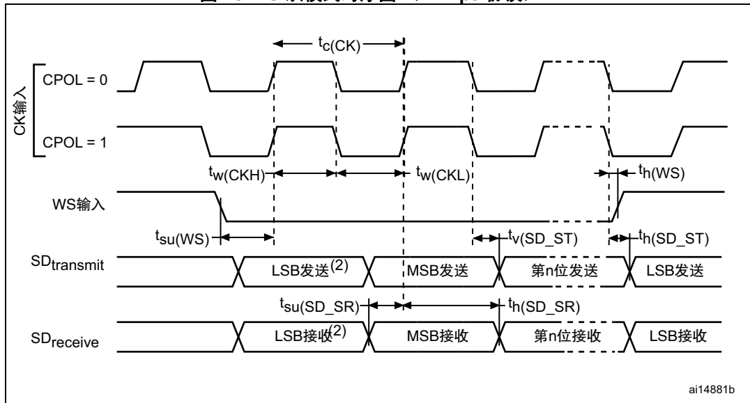
图 28. I 2 S 从模式时序图 (Philips 协议) (1)
