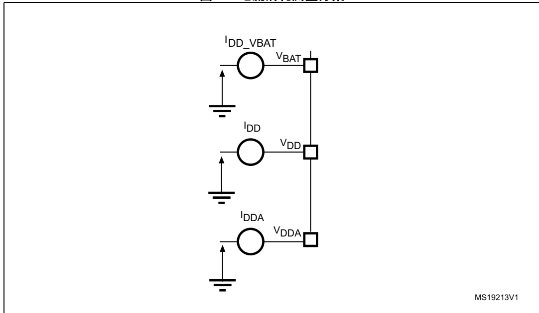
图 12. 电流消耗测量方案
