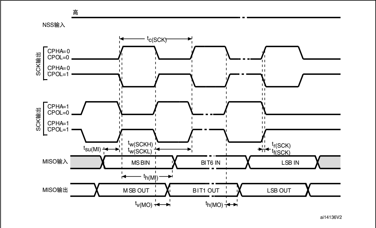
图 27. SPI 时序图 – 主模式 (1)
