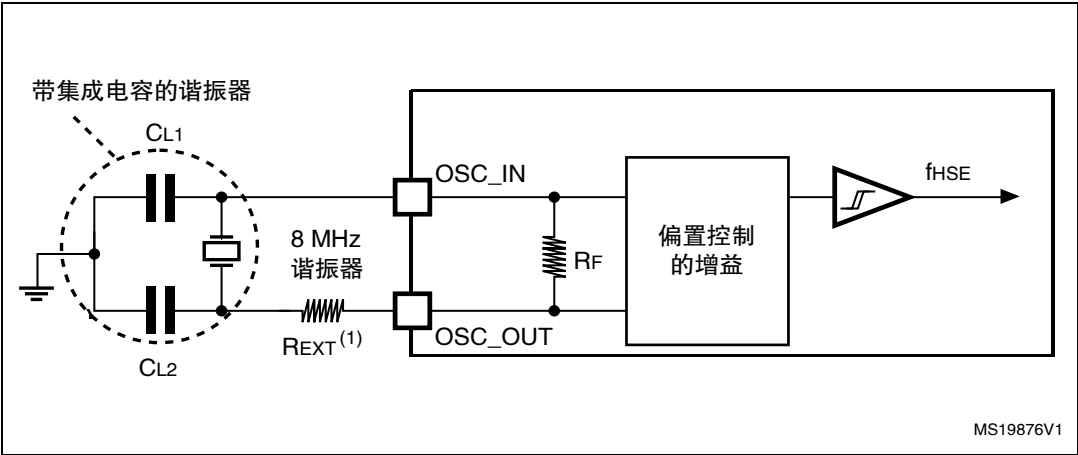
图 16. 采用 8 MHz 晶振的典型应用
