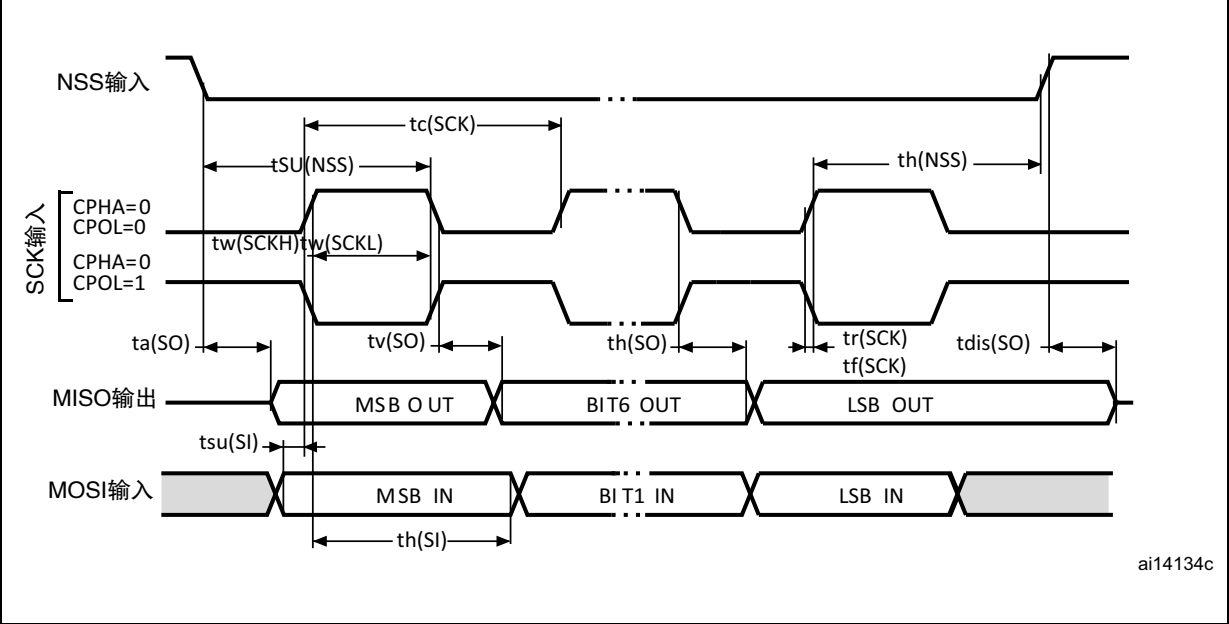
图 25. SPI 时序图 – 从模式且 CPHA = 0
