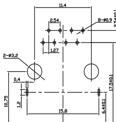
P. C. B参考图
