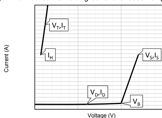
Fig.4 - VI Curve
