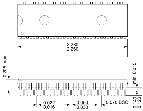
64SDIP
