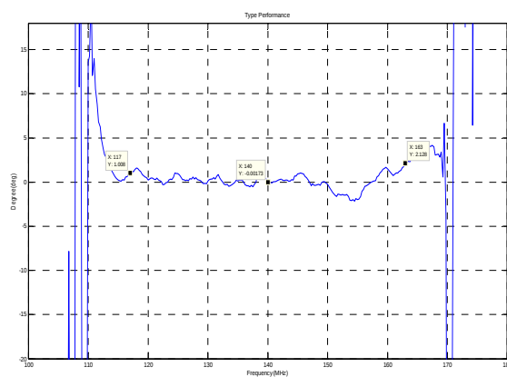
Phase Linearity( f_0 \pm 23\text{MHz} )
