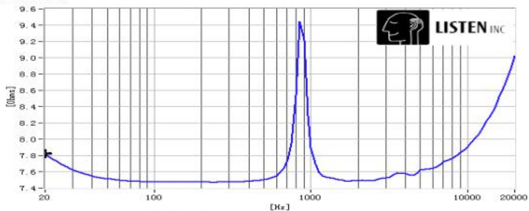
阻抗曲线
