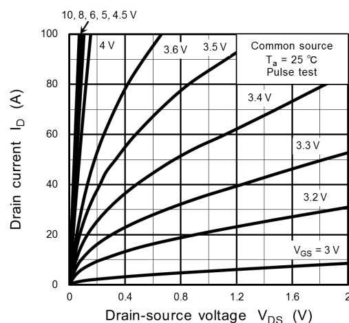
Fig. 8.2 I_D - V_{DS}
