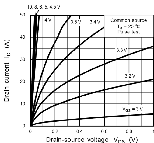
Fig. 8.1 I_D - V_{DS}
