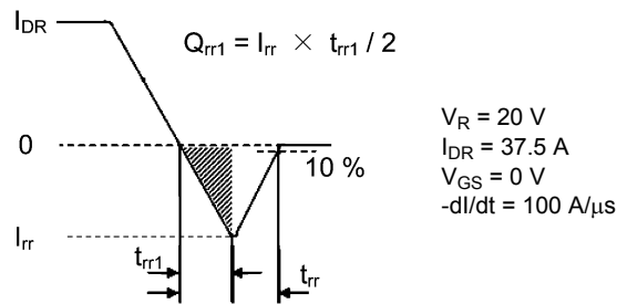
Fig. 6.4.1 t rr Waveform
