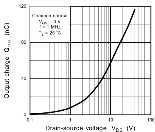
Fig. 8.12 Q_{oss} - V_{DS}
