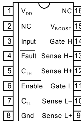
SOIC Package (WM)
