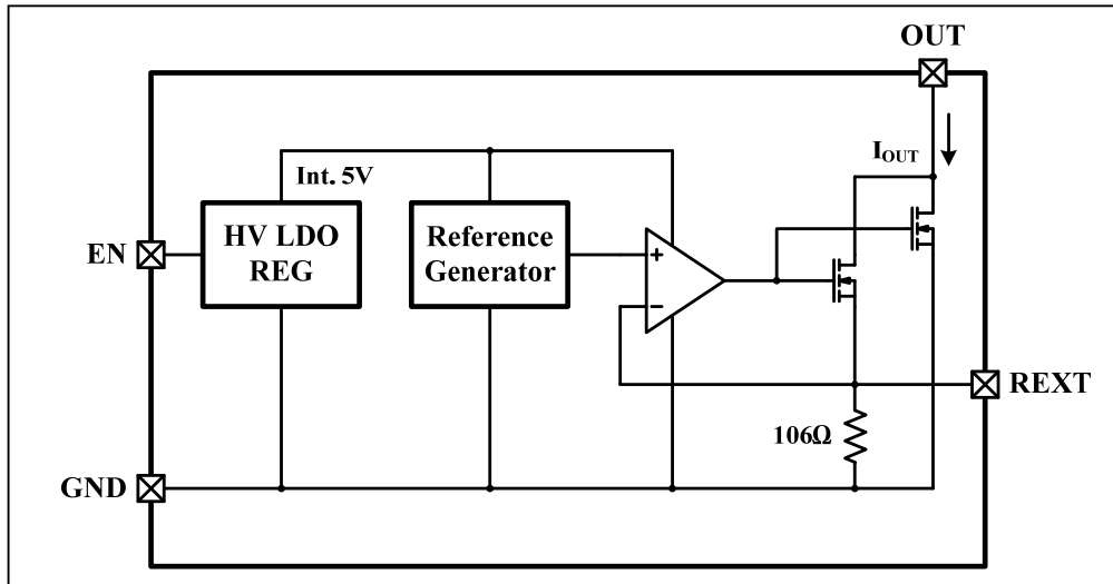
IS32LT3170
