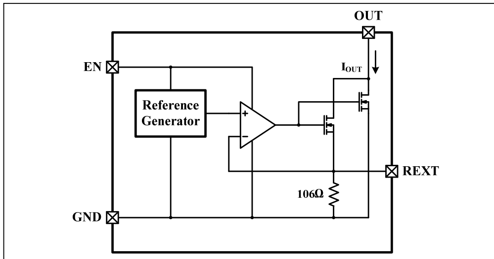
IS32LT3171
