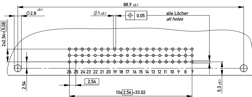
Leiterplatten-Lochbild / PCB drillhole pattern
