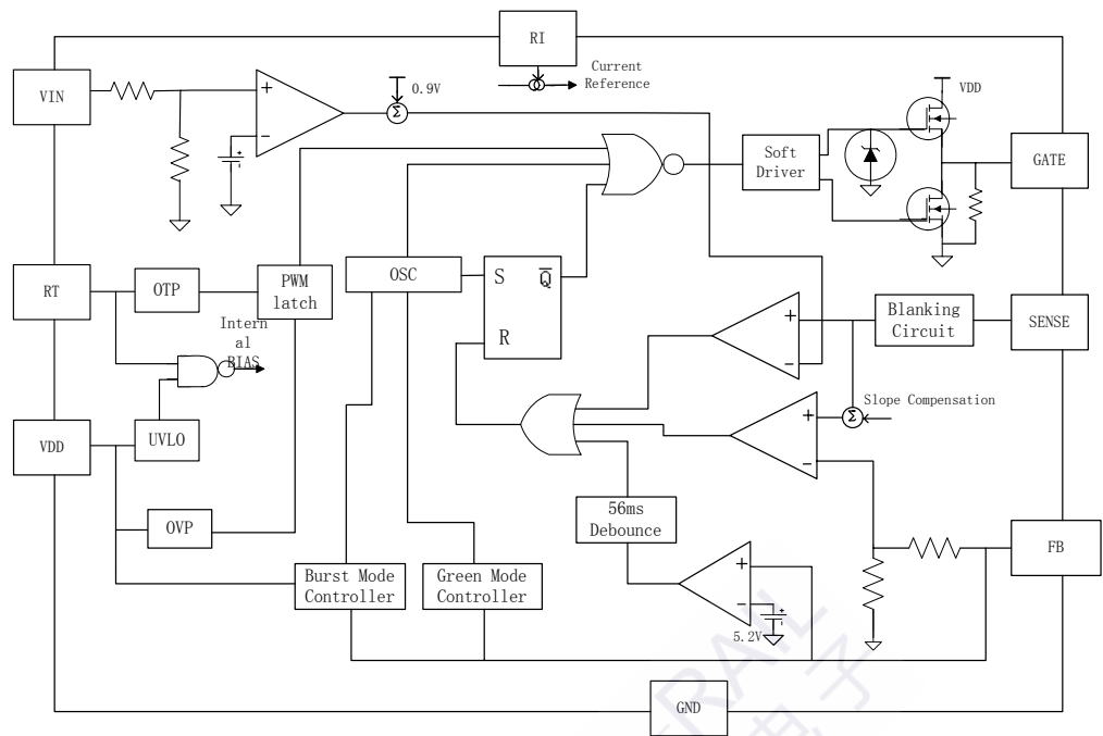
功能框图
