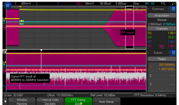
그림 21d: 검색 lister 디스플레이에 표시되어 있듯이 RF 신호는 200 MHz에서 안정적으로 유지됩니다.
