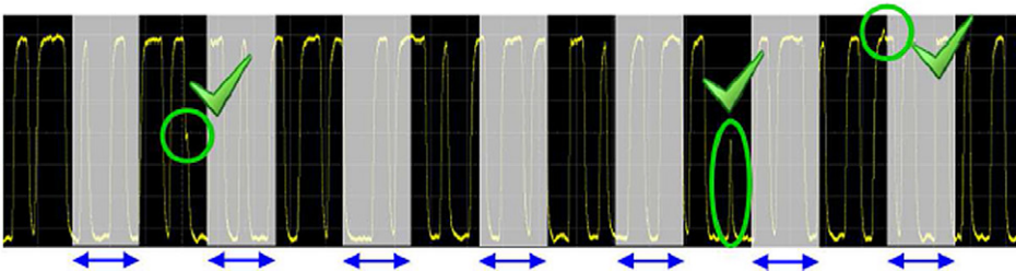
그림 10: InfiniiVision 30000T X-시리즈는 초당 100만 개의 파형을 지원합니다. 데드 타임이 짧기 때문에 간헐적 이벤트를 캡처할 수 있는 확률이 높습니다.
