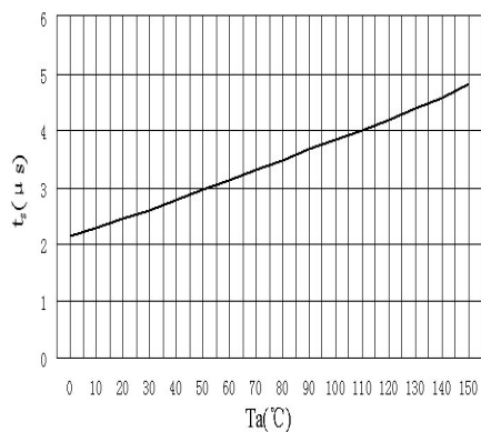
t_s-T_a
