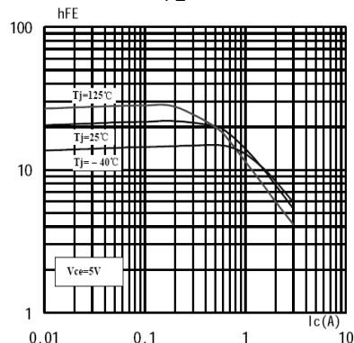
h_{FE}-I_C
