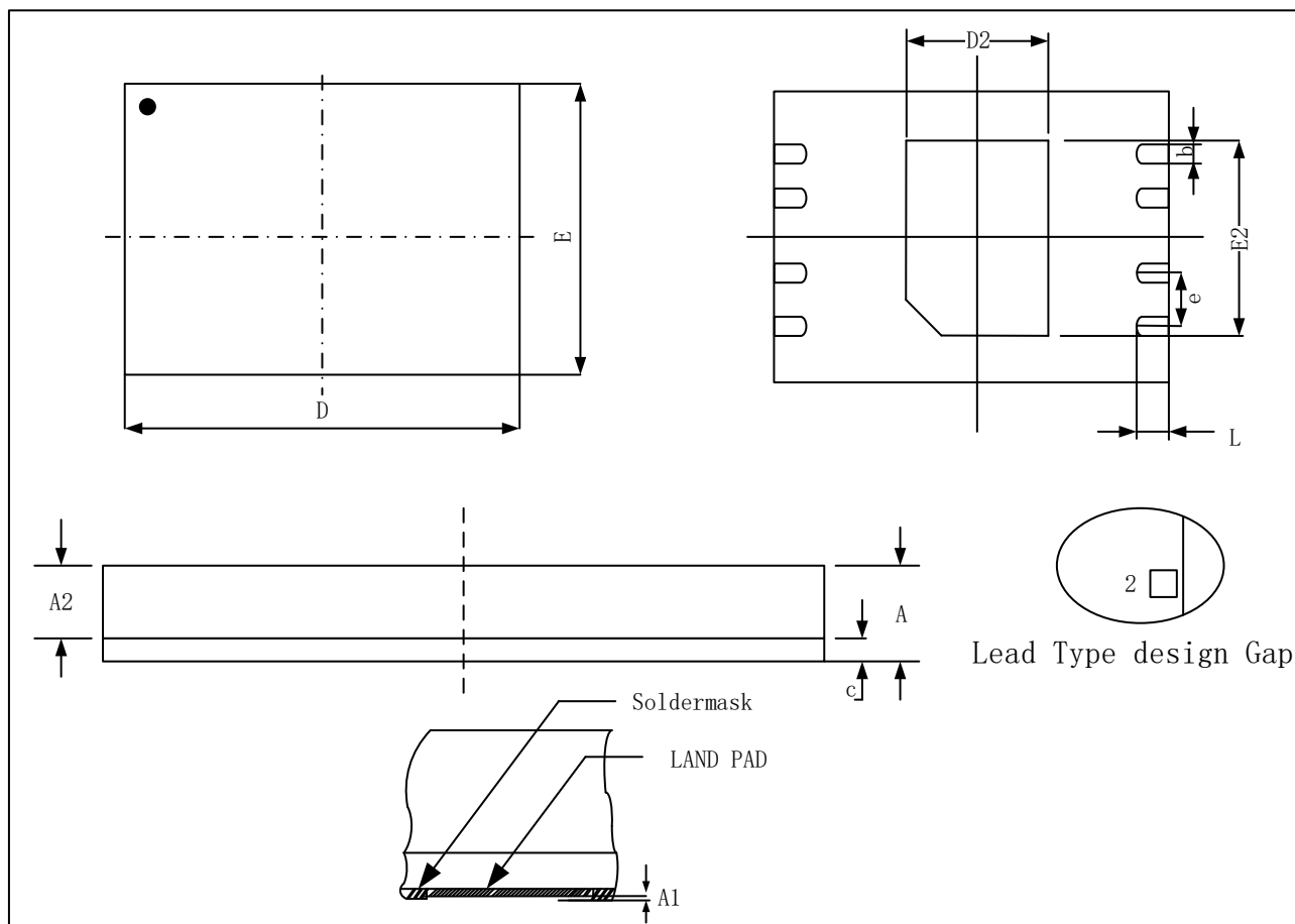
Figure22-4. GD Type1 LGA8 (6*8 mm)
