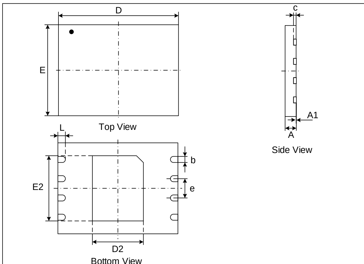
Figure22-1. WSON8 (8*6mm)
