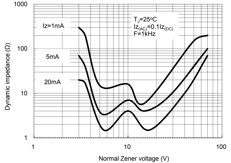
Fig. 2 Effect of Zener voltage on Zener impedance
