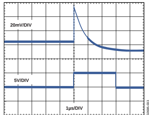
图32. 中间电平毛刺能量, 代码0x80至0x7F
