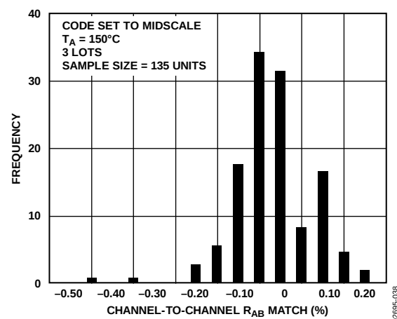
图37. 通道间电阻匹配(AD5262)
