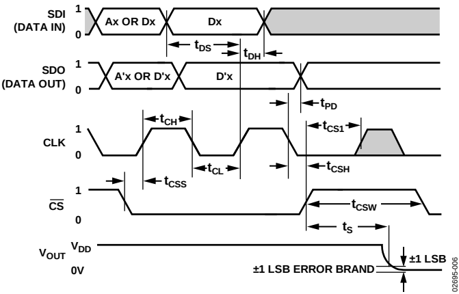
图5. 详细时序图
