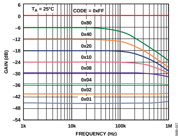
图26. 增益与频率和代码的关系, R_{\text{AB}} = 50 \text{ k}\Omega
