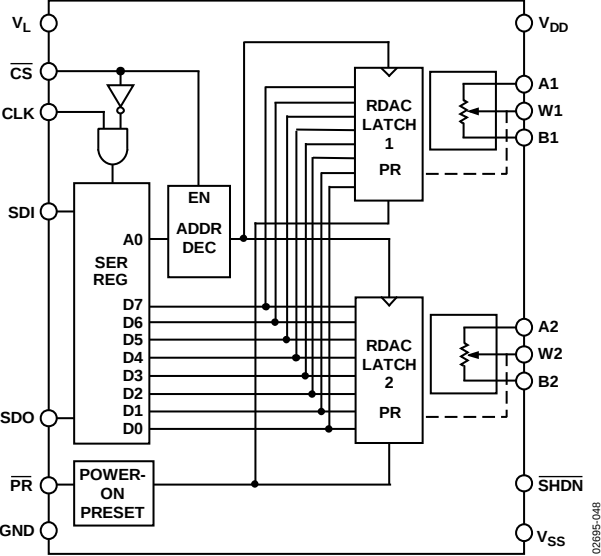
图47. AD5262功能框图
