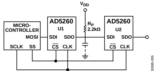
图 52. 菊花链配置
