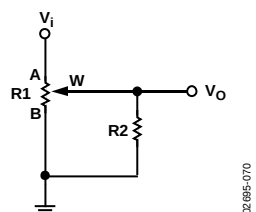
图70. 利用对数调整特性调节电阻
