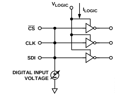
图45. V_{LOGIC} 电流与数字输入电压的关系
