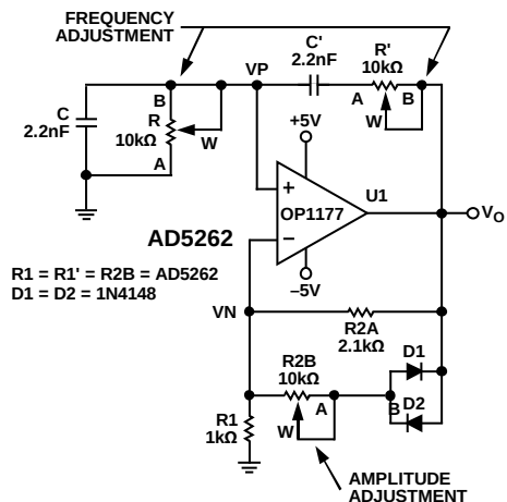
图67. 带幅度控制的可编程振荡器
