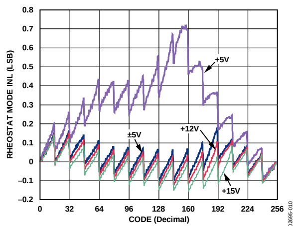
图9. R-INL与代码和电源电压的关系
