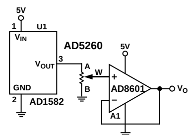
图60. 可编程基准电压源
