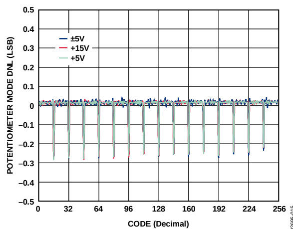
图14. DNL与代码和电源电压的关系
