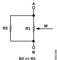
图69. 降低标称电阻
