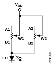
图68.利用线性调整特性将电阻值减半
