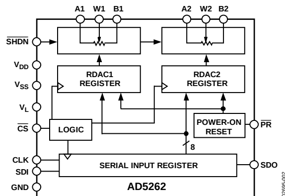
图2. AD5262
