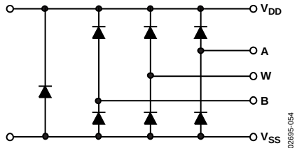
图56. 由 V_{DD} 和 V_{SS} 设置的最大端电压
