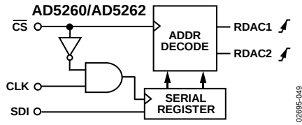
图 48. 等效输入控制逻辑
