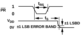
图6. 预设时序图
