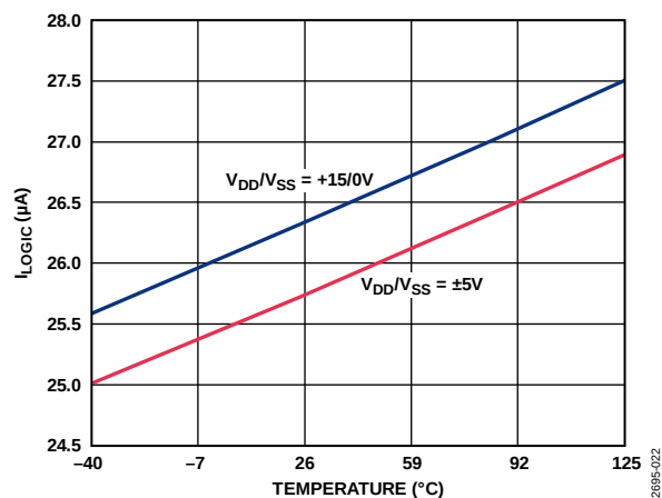
图21. I_{\text{LOGIC}} 与温度的关系
