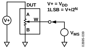
图38. 电位分压器非线性误差 (INL, DNL)
