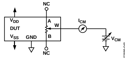
图44. 共模漏电流
