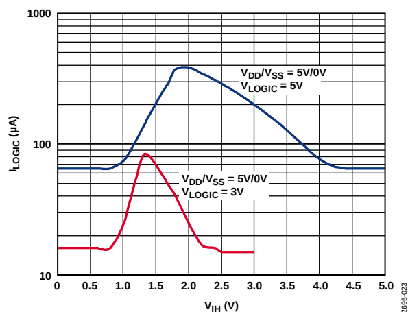
图22. I_{\text{LOGIC}} 与数字输入电压的关系
