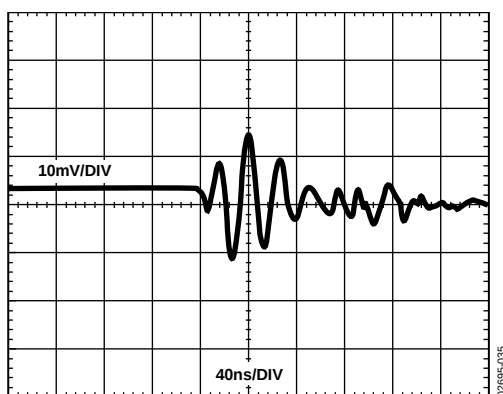
图34. 数字馈通与时间的关系
