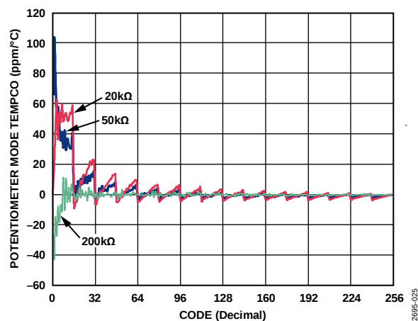
图24. 电位计模式温度系数 \Delta V_{\text{WB}}/\Delta T 与代码的关系
