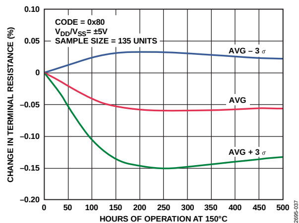
图36. 长期电阻漂移
