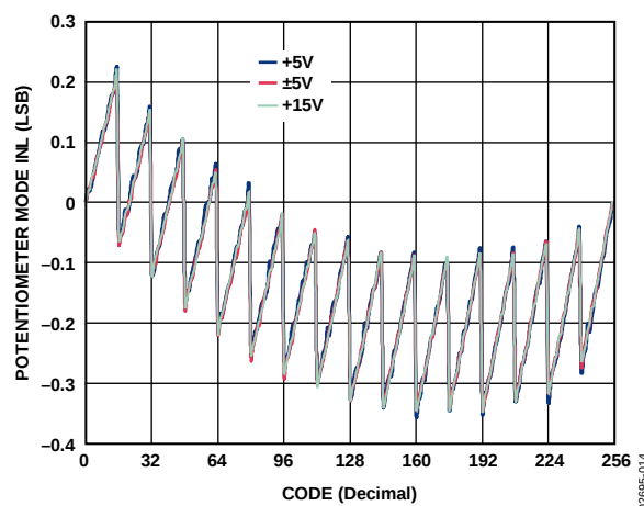
图13. INL与代码和电源电压的关系
