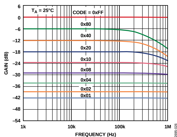
图25. 增益与频率和代码的关系, R_{\text{AB}} = 20 \text{ k}\Omega
