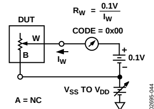
图43. 增量导通电阻
