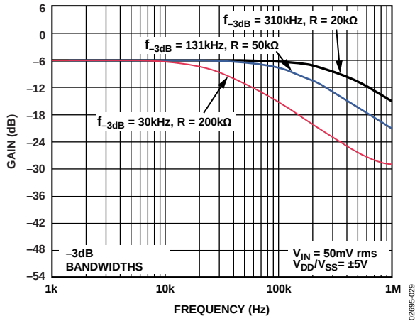
图28. -3 dB带宽
