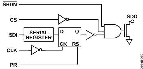
图 49. AD5260的SDO输出详细原理图
