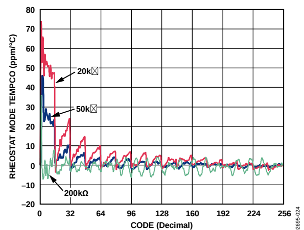
图23. 可变电阻器模式温度系数 \Delta R_{\text{WB}}/\Delta T 与代码的关系
