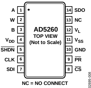
图7. AD5260引脚配置
