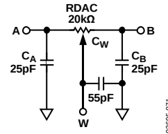
图57. RDAC电路仿真模型(RDAC 20 k \Omega )
