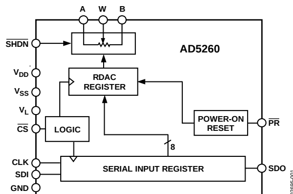
图1. AD5260
