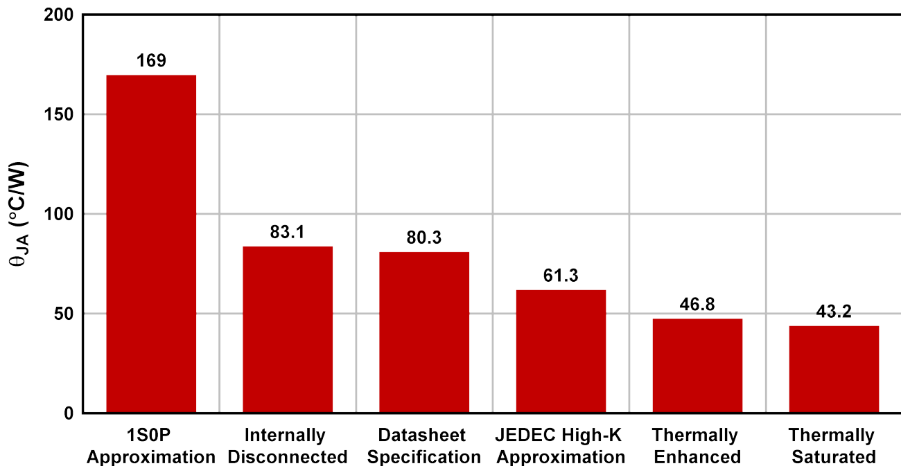
图 8-8. TPS746-Q1 (WSN) R_{\theta JA} vs Board Layout
