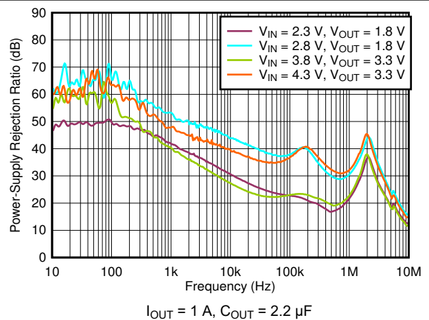
图 6-36. PSRR vs Frequency
