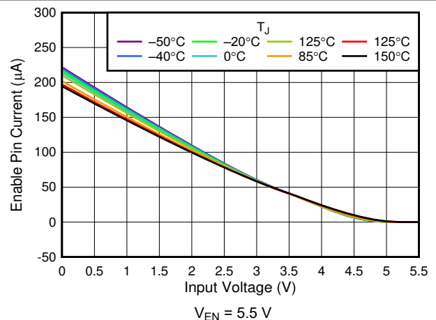
图 6-22. I_{EN} vs V_{IN}
