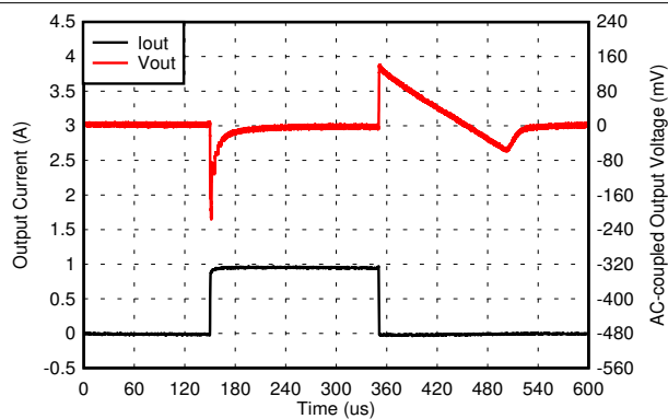
图 6-26. 1-mA to 1-A Load Transient (0.55 V)
