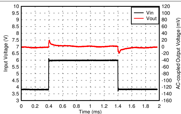
图 6-25. 3.3-V Line Transient
