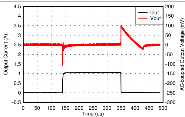
图 6-26. 1-mA to 1-A Load Transient (0.55 V)
