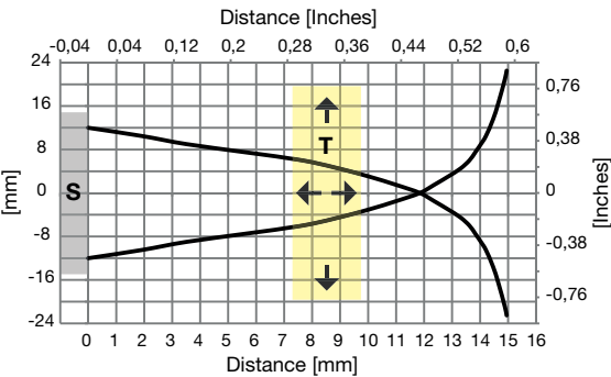
Fig. 5 M30 Flush
