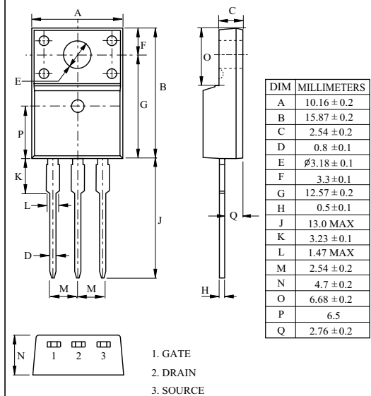
KHB7D0N65F1
