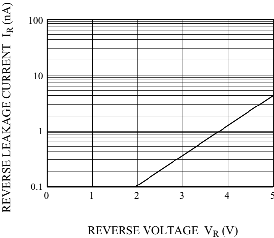
I_R - V_R
