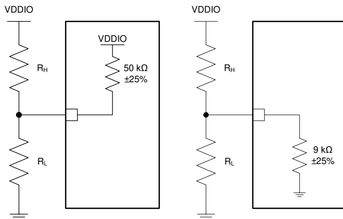
图 8-10. Bootstrap Circuits
