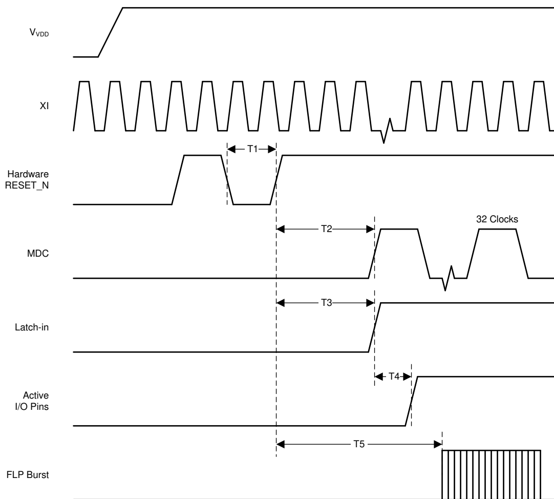
图 7-3. Reset Timing
