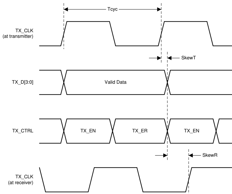
图 7-11. RGMII Transmit Timing
