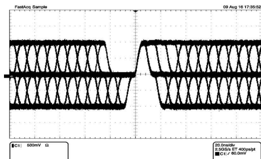
mV per Div 500 mV nS per Div 20 ns 图 7-18. 100BASE-TX PMD Eye Waveform
