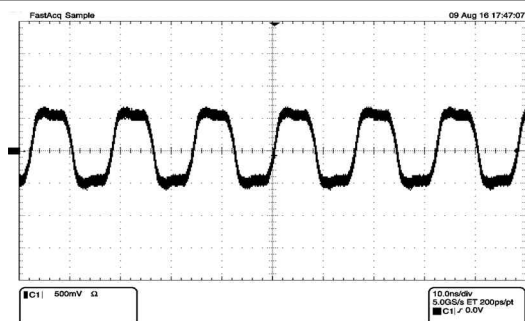
mV per Div 500 mV nS per Div 10 ns 图 7-20. 100BASE-FX Waveform
